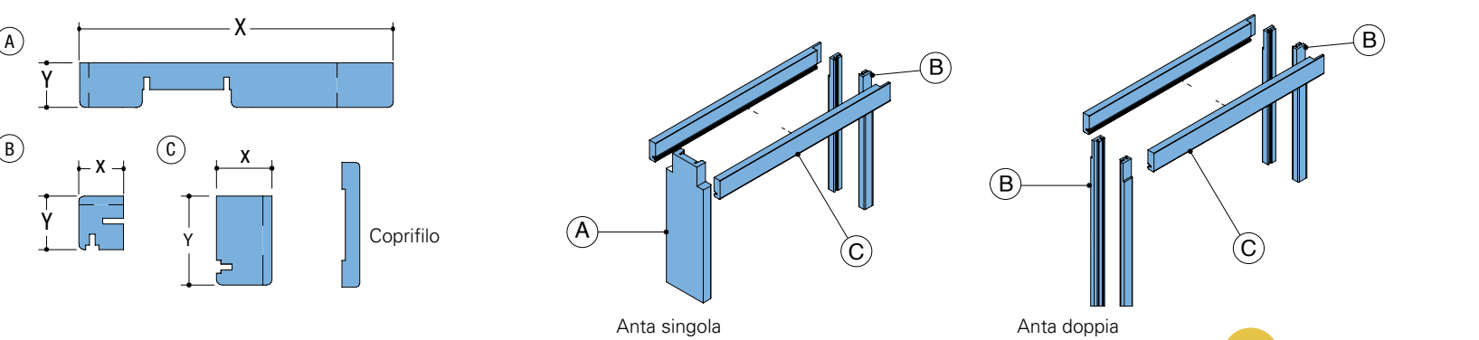
ANTA SINGOLA Cod. ACC.463 SF Senza fresata
