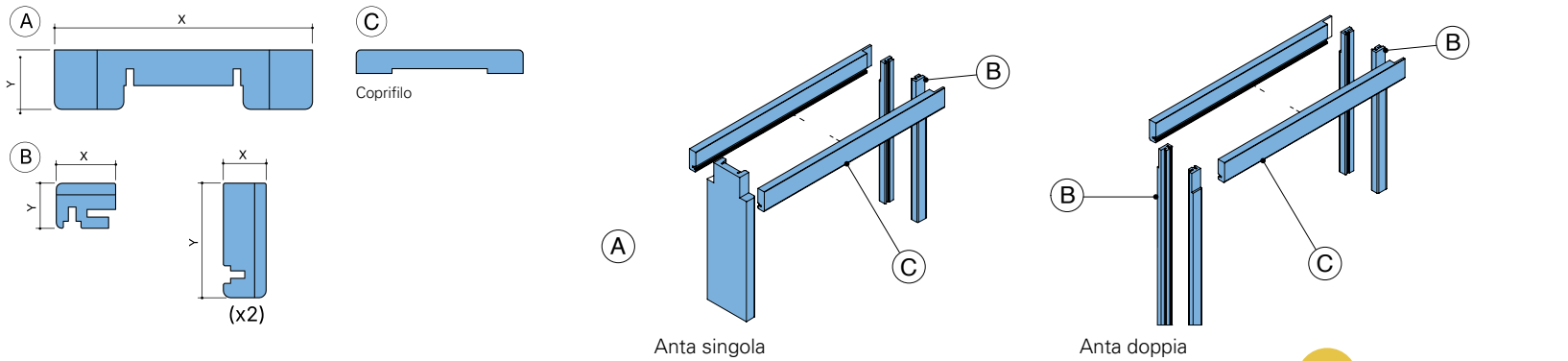
ANTA SINGOLA Cod. ACC.461 SF Senza fresata
